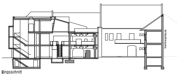
längsschnitt
