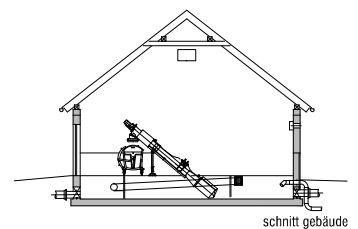
schnitt gebäude
