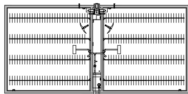
reinigungsbecken (sbr-anlage)
